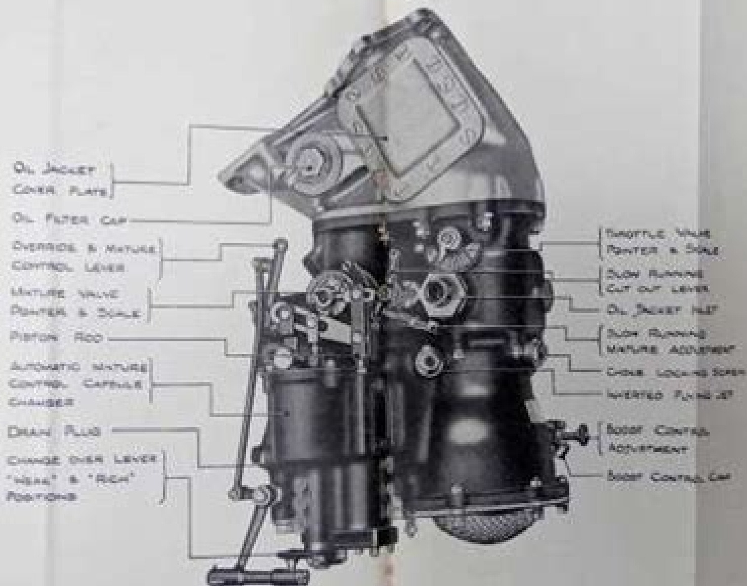
CLAUDE L. HOBSON A.V. 70 M. CARBURETTOR
