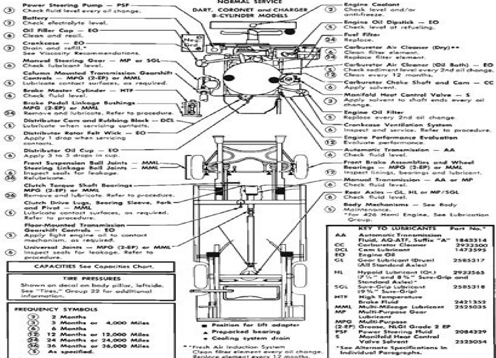
Fig. 2—Lubrication Chart
