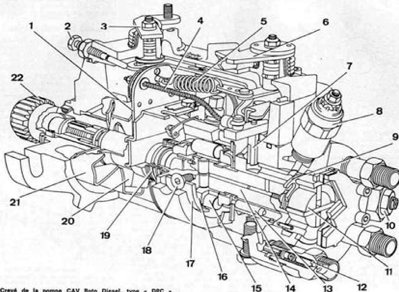
Crevé de la pompe CAV Roto Diesel, type - DPC -
