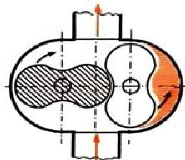
Máquina soplane capsular.
