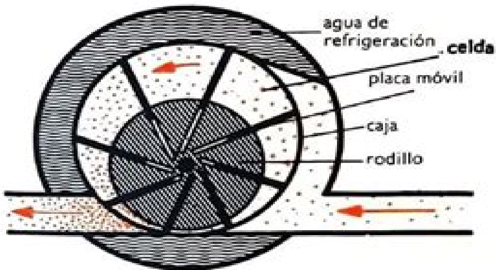
Compresor rotativo.
