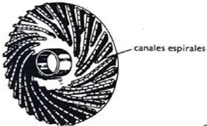
Interior de un rodete.
