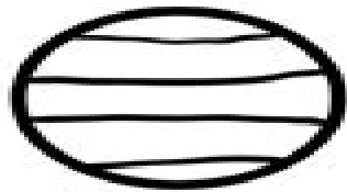
Venus
