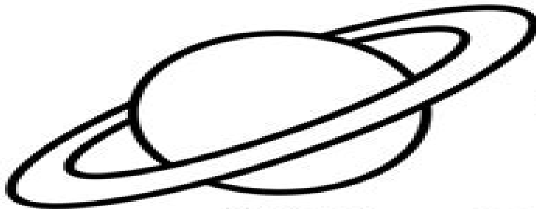
Uranus
