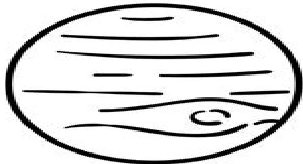
Jupiter
