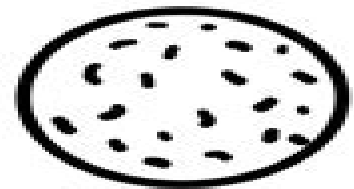
Mars
