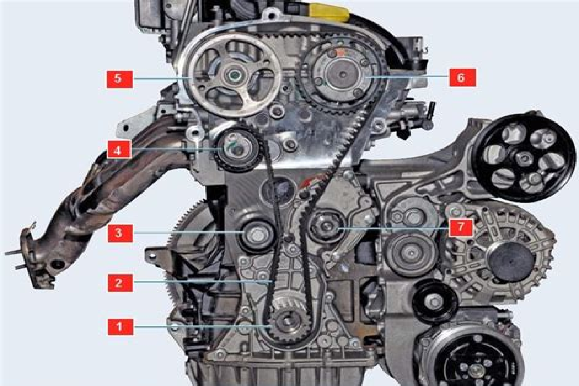
Привод ГРМ двигателя F4R: 1 - зубчатый шкив коленчатого вала; 2 - ремень привода ГРМ; 3 - опорный ролик ремня; 4 - натяжной ролик ремня; 5 - зубчатый шкив распределительного вала выпускных клапанов; 6 - исполнительный механизм системы изменения фаз газораспределения; 7 - шкив насоса охлаждающей жидкости
