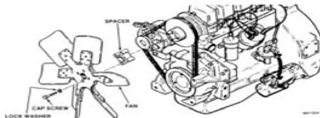
Fan Installation
