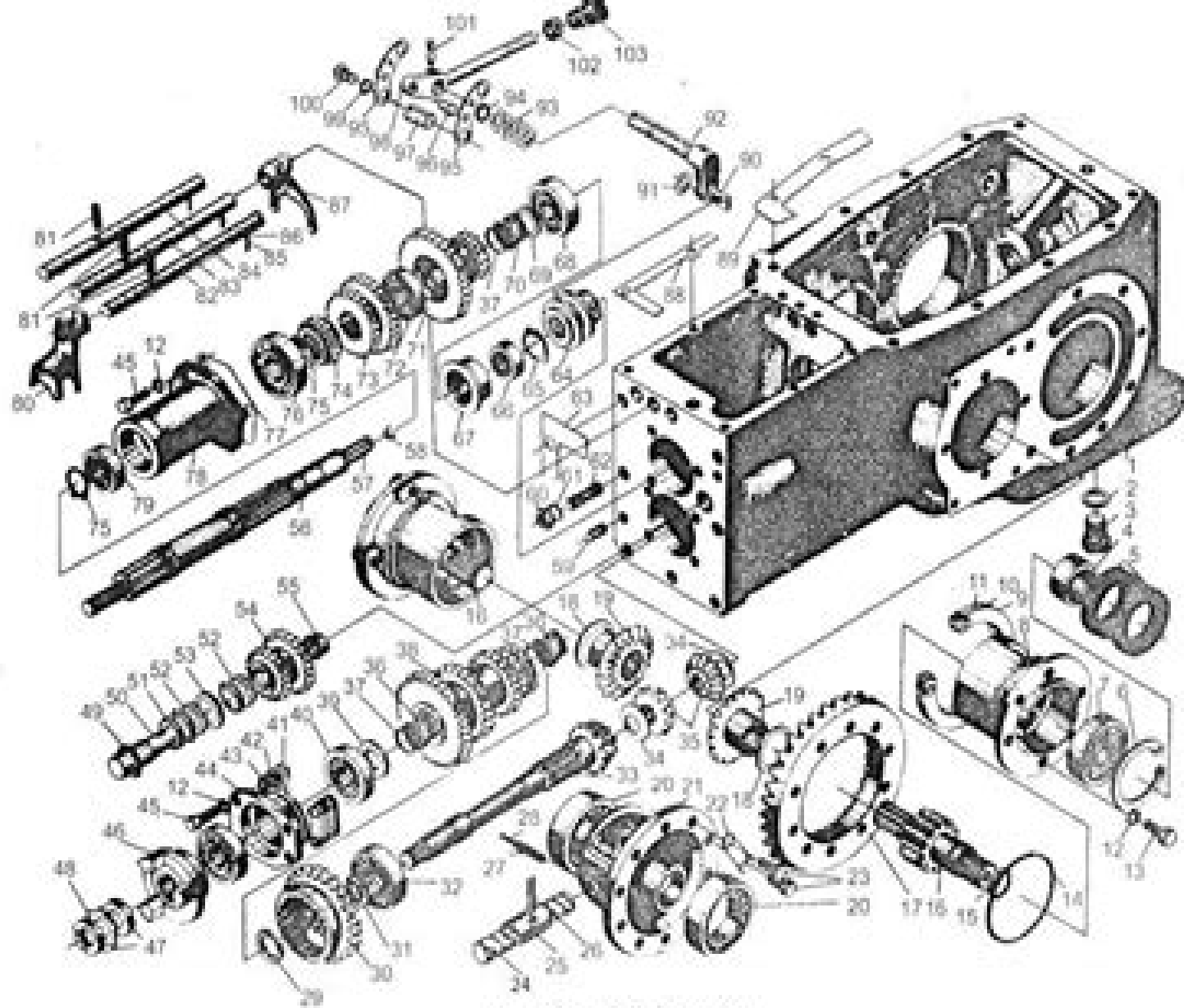
图9. 传动箱总成(双速)
