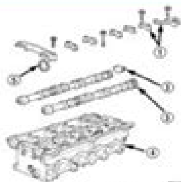
Fig. 16 Camshafts
